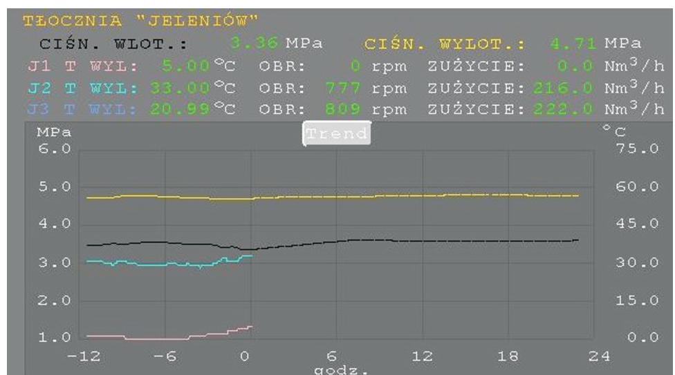
Rys. 4. Grafika szczegółowa dla tłoczni w Krzywej. Odnotowane i zaplanowane ciśnienia dolotowe i wylotowe tłoczni oznaczono na wykresie liniami czarną i żółtą. Pozostałe linie oznaczają odnotowane temperatury wylotowe gazu dla poszczególnych sprężarek (wartość „0” związana jest z aktualnym brakiem danych)
